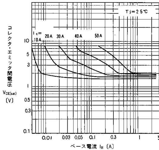
出力特性
