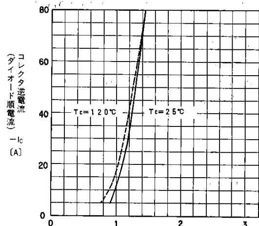
エミッタ・コレクタ間電圧 V_{ECO} (V) (ダイオード順電圧) 高速フリーホイリングダイオード順電圧
